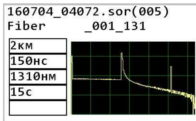
Рис. 20 Сохранённая рефлектограмма
