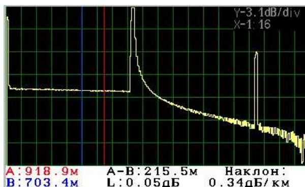
Рис. 12 Просмотр рефлектограммы.
